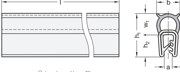
Üst sızdırmazlık profili
